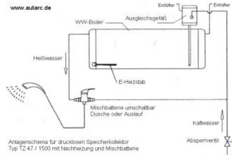
Bildbeispiel Modell Variante TZ47/1500/20_200 mit 20 Röhren ( 2,5 m 2 ) und 200 Liter WW-Boiler
