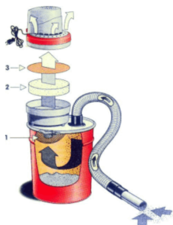
Aschesauger kpl. mit Motor und 3-fach Filter
